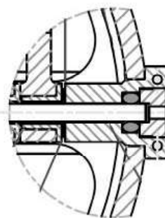
DETAIL C-C SCALE: 4/1
